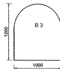
B3 Glas 6 mm stark
