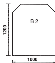
B2 Glas 6 mm stark
