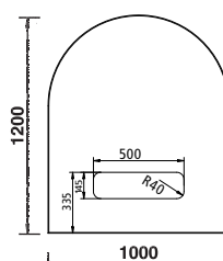
B3 Glas 6 mm stark mit Ausschnitt
