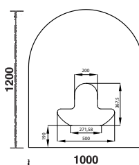
B3 Glas 6 mm stark für Anschluss unten
